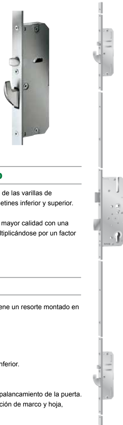
Varillas de transmisión redondas
